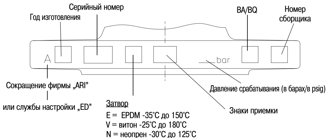
Рис. 4: Корпус (фланец на выходе)
